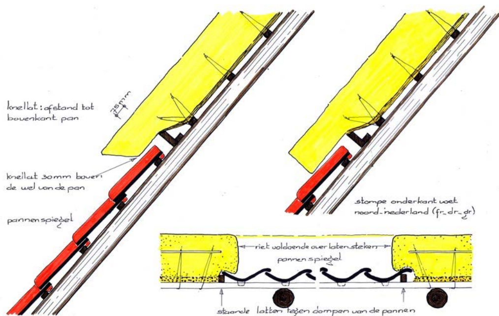
Figuur 9: Aanbrengen pannenspiegel
