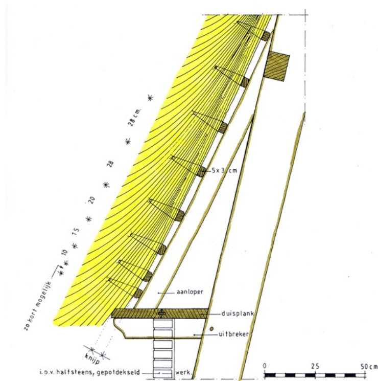
Figuur 20: Detaillering dakvoet met duisbord of duisplank
