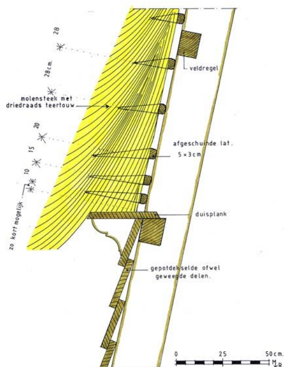
Figuur 21: Detaillering dakvoet met duisplank bij gepotdekselde wanden
