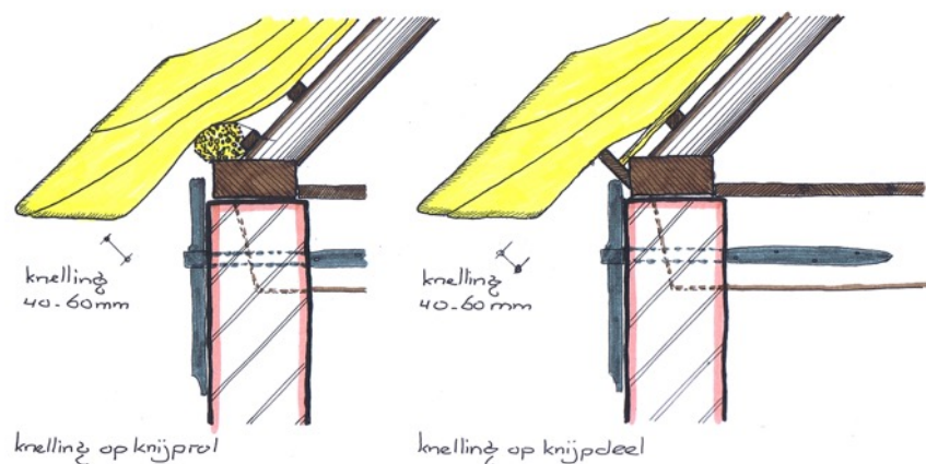
Figuur 2: Voorbeeld van knelling op een knijplank of een knijprol bij traditioneel dekken. Dezelfde knelling geldt bij toepassing van een onderplaat en het toevoegen van isolatie.
