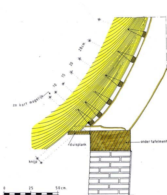
Figuur 22: Detaillering dakvoet met duisplank bij gemetselde onderzijde
