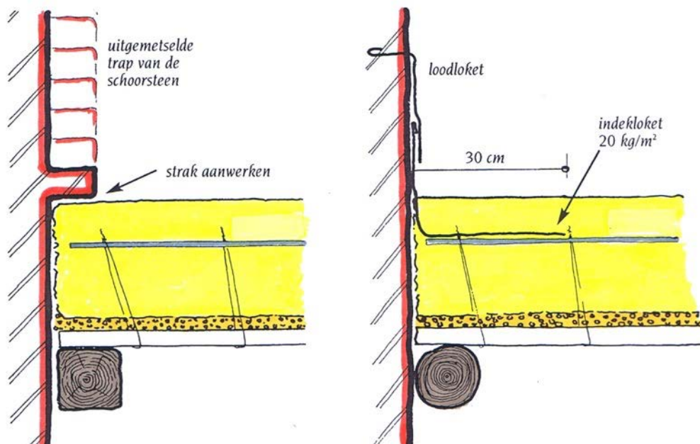
Figuur 10: Aansluiting op muurwerk zonder en met loketten
