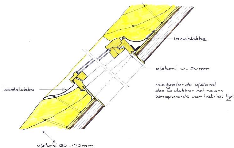
Figuur 14: Aanbrengen dakraam in rietbedekking
