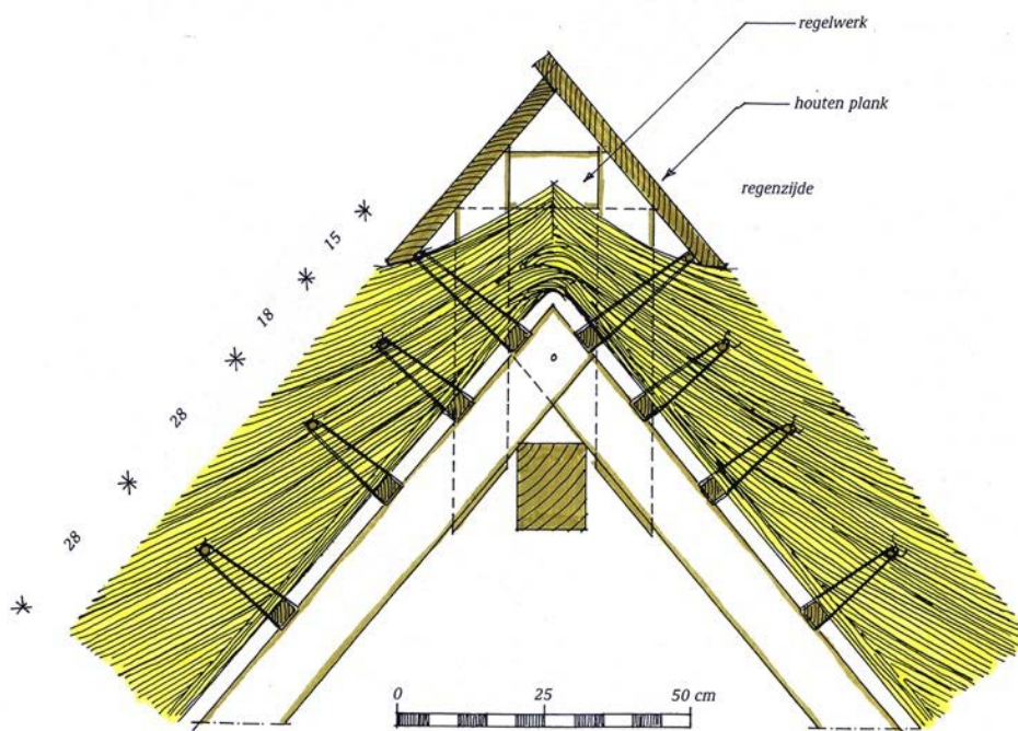
Figuur 8: Aanbrengen van houten nokafdekking
