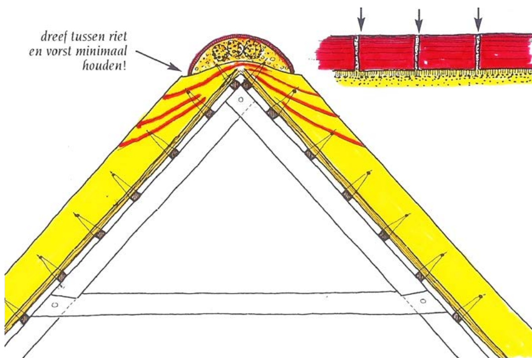
Figuur 6: Doorsnede nok sporenkap met rietvorsten.
