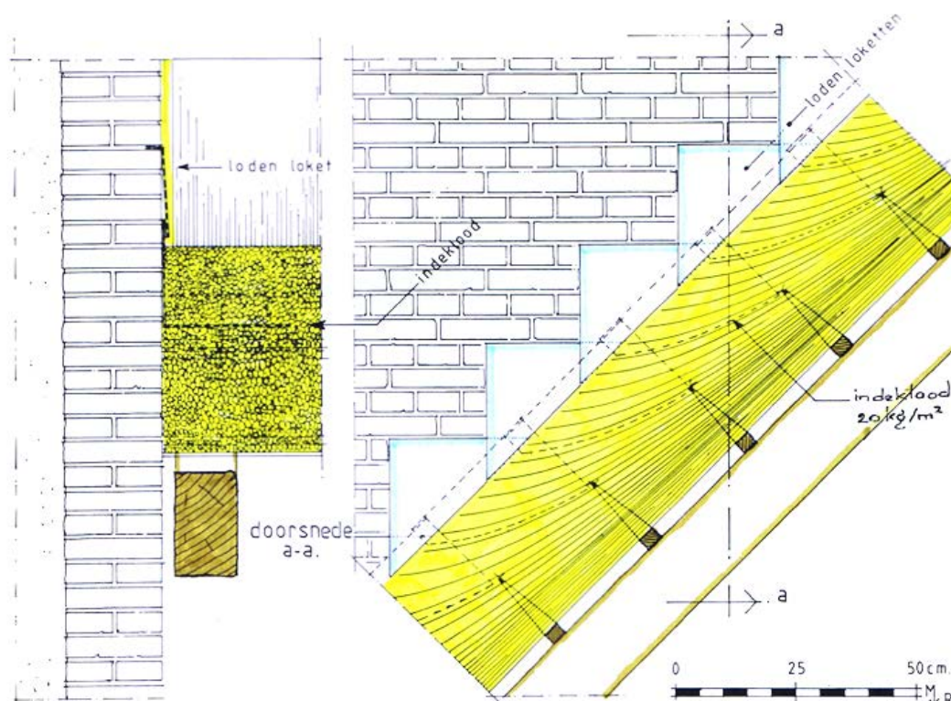
Figuur 11: Aanbrengen loodloketten
