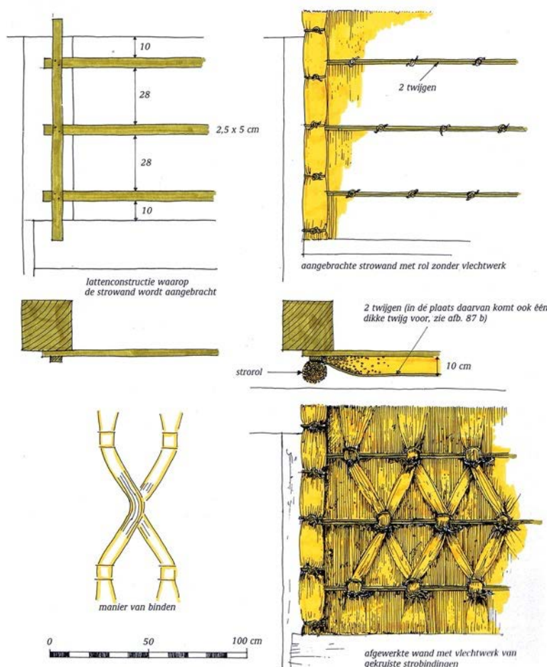
Figuur 15: Aanbrengen siervlechtwerk op wanden
