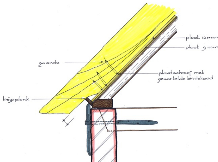
Figuur 17: Dakvoet met de opbouw van een stromingsdichte onderschil met plaatmateriaal van 12 mm, respectievelijk 9 mm.
