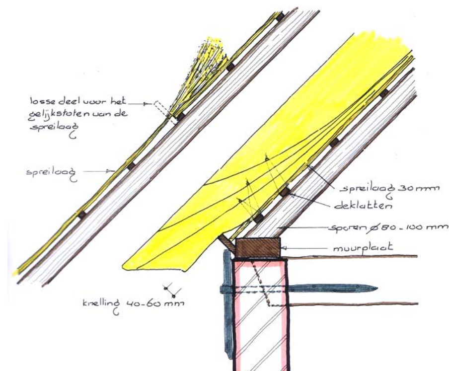
Figuur 4: Opbouw rietbedekking aan dakvoet - aanbrengen spreilaag.
