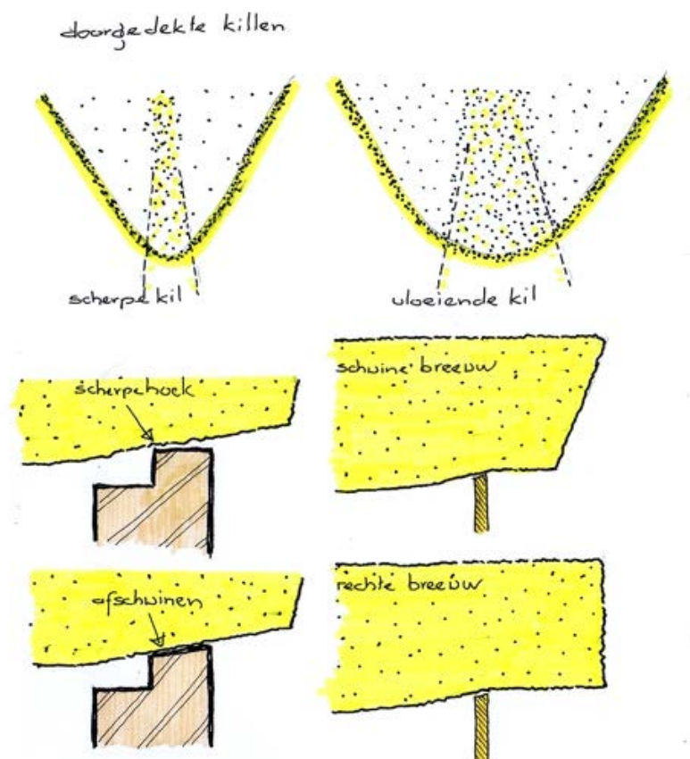
Figuur 3: Voorbeelden van een scherpe kil en een vloeiende kil. Detaillering van een (streekgebonden) rechte of schuine breeuw.
