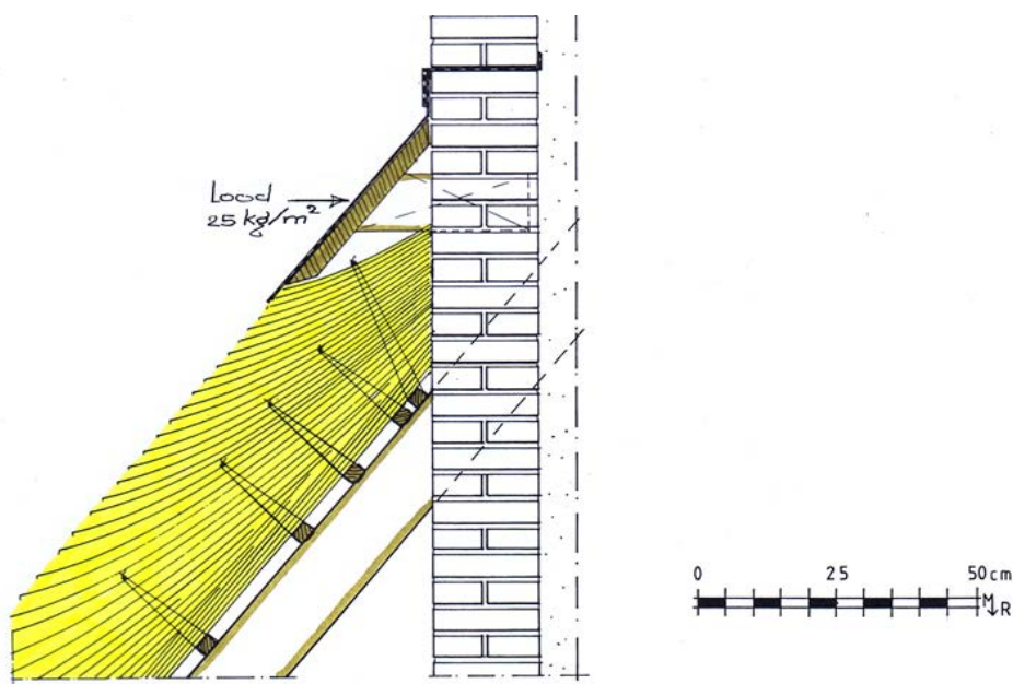
Figuur 12: Aansluiting riet bij opgaand metselwerk
